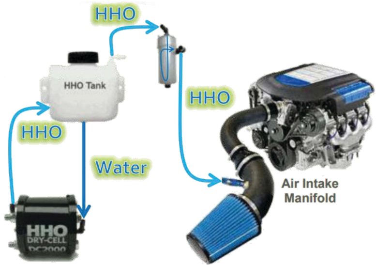
Schema di collegamento dei componenti
